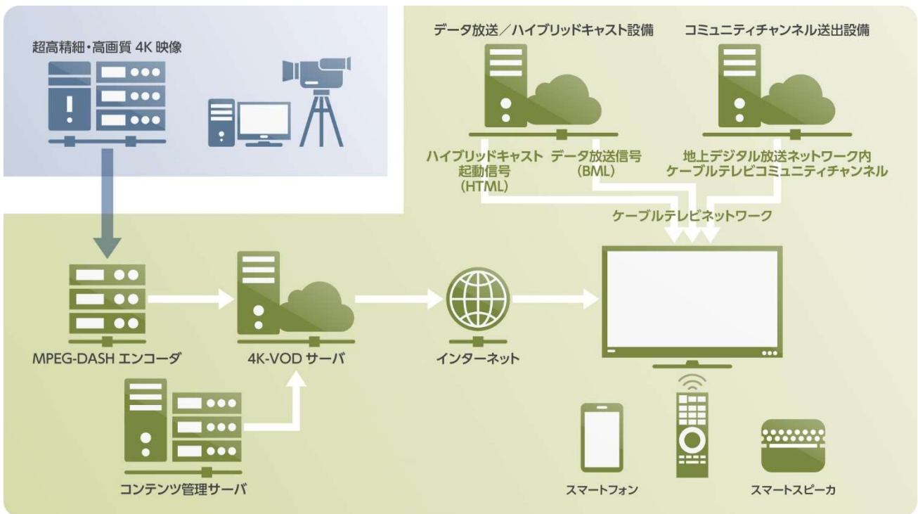
ケーブルテレビハイブリッドキャストを利用した場合のシステムイメージ
